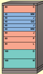
275 compartimientos en 11 gavetas No. 240-680-1020 No. 241-680-1020
