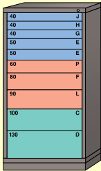
210 compartimientos en 10 gavetas No. 240-680H No. 241-680H
