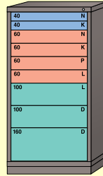
144 compartimientos en 9 gavetas No. 240-680-1013 No. 241-680-1013
