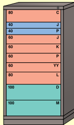
163 compartimientos en 10 gavetas No. 240-680-1021 No. 241-680-1021
