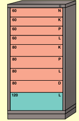
140 compartimientos en 9 gavetas No. 240-680-1012 No. 241-680-1012
