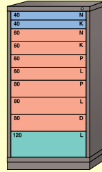
164 compartimientos en 10 gavetas No. 240-680-1010 No. 241-680-1010
