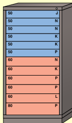
240 compartimientos en 12 gavetas No. 240-680-1005 No. 241-680-1005
